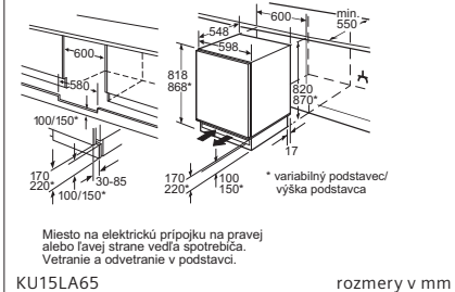
Chladiaci automat
