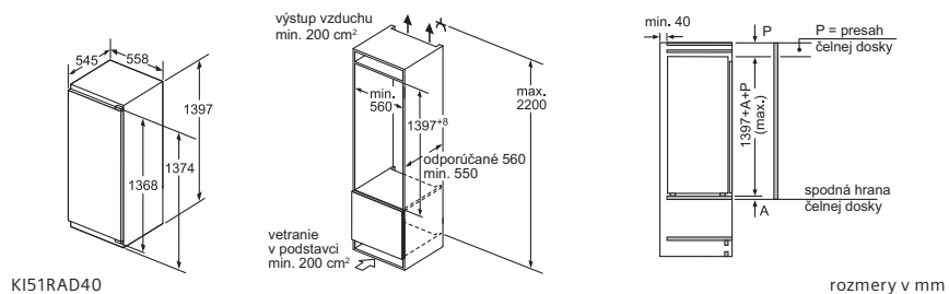
Chladiaci automat
