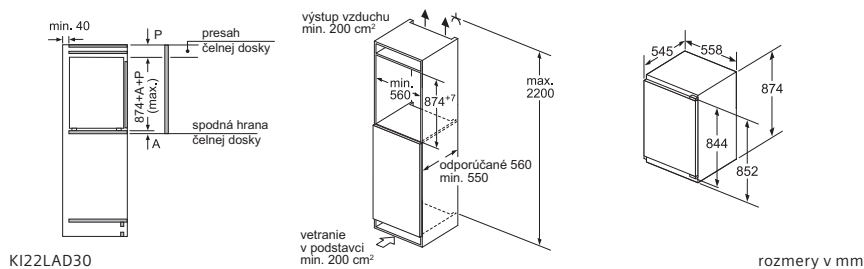
Chladiaci automat
