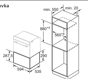
Ohrevná zásuvka
