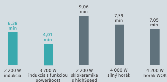
Čas potrebný na ohrev 2 litrov vody s teplotou 15 °C na teplotu 90 °C (v minútach)
